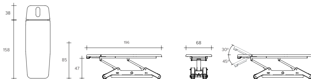
DIMENSIONES DEL PRODUCTO (cm)
